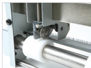
Unité de perforation longitudinale, complète, partielle ou séquentielle.
